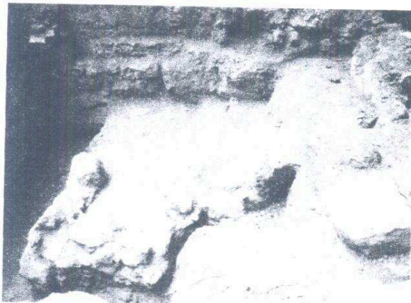
Subestructura Norte E-4
